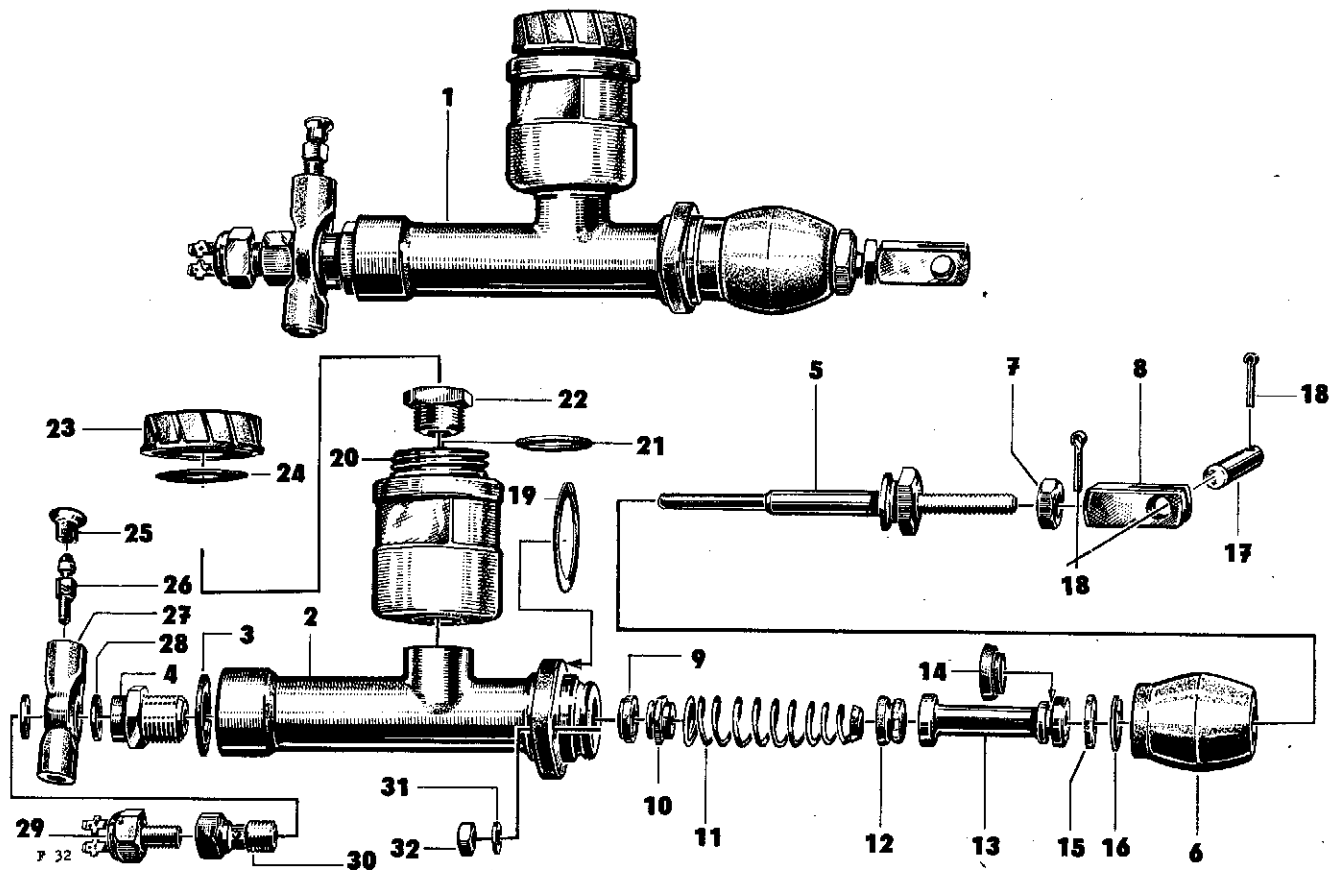
Hauptbremszylinder - Master brake cylinder
