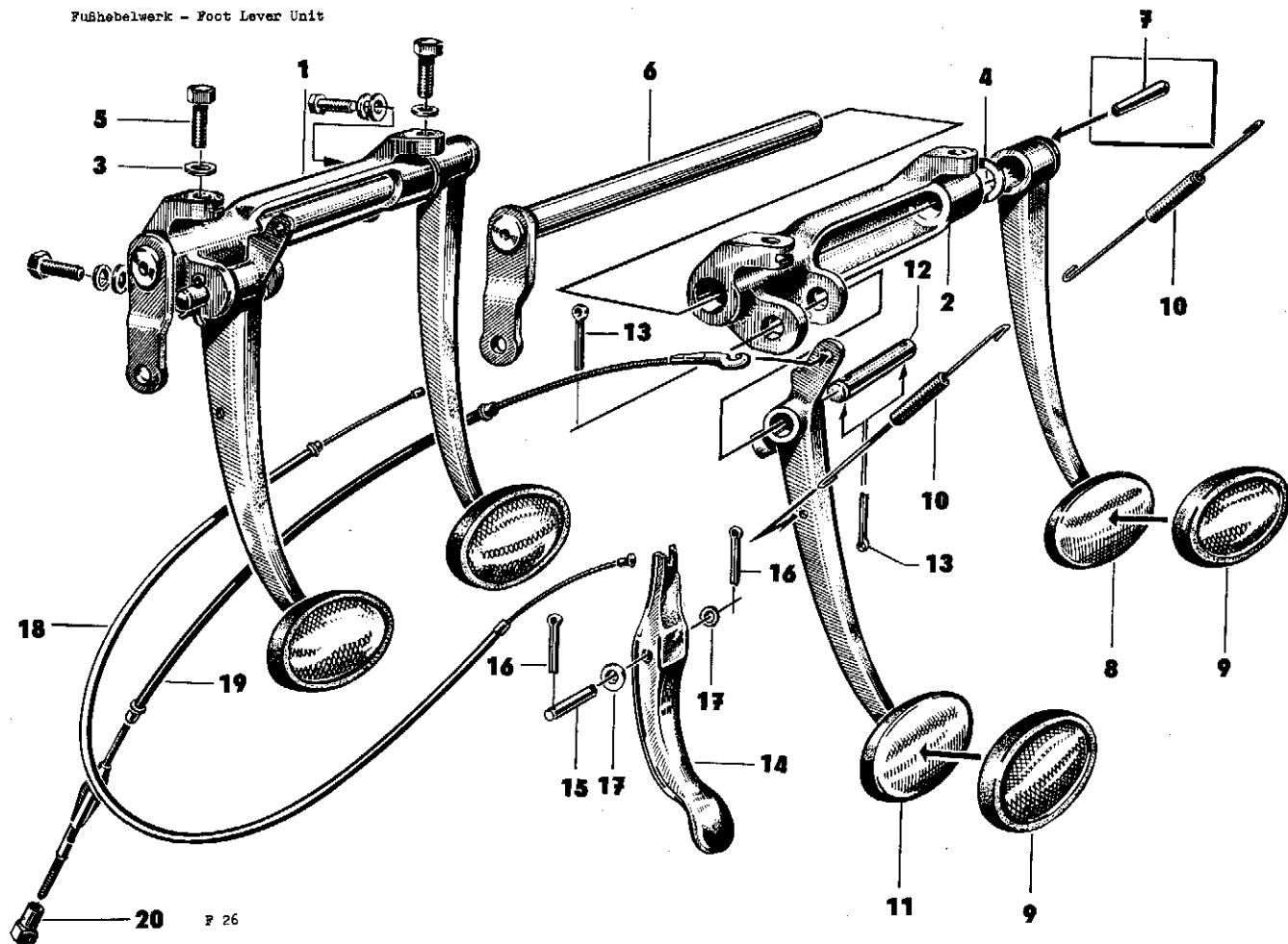
Fußhebelwerk - Foot Lever Unit
